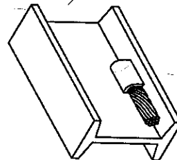
SOLDADURA CADWELD TIPO ST
