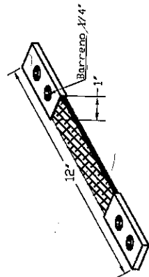
CONECTOR DE COBRE TRENZADO FLEXIBLE TIPO BD
